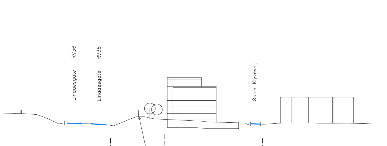
Snitt 1
